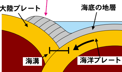
海底の地層が大陸にくっつく過程
