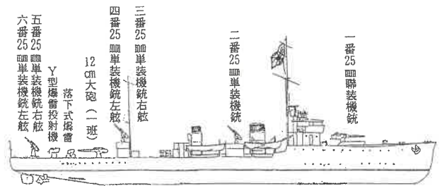
山田湾に配備されていた第一号掃海艇の側面図。長さ76.2メートルで97人が乗り組んでいました。
